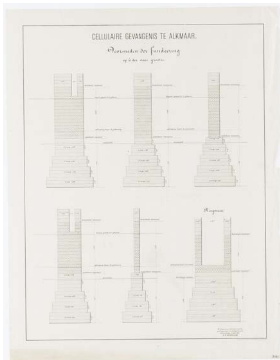
Links: Bouwtekening J.F. Metzelaar juli 1883 fundering (Regionaal Archief Alkmaar)
