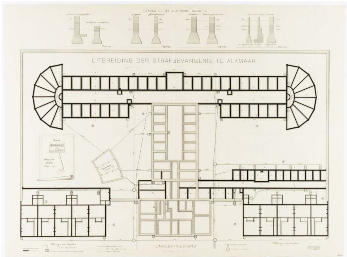
Bouwtekening uitbreiding W.C. Metzelaar september 1891 fundering (Regionaal Archief Alkmaar)
