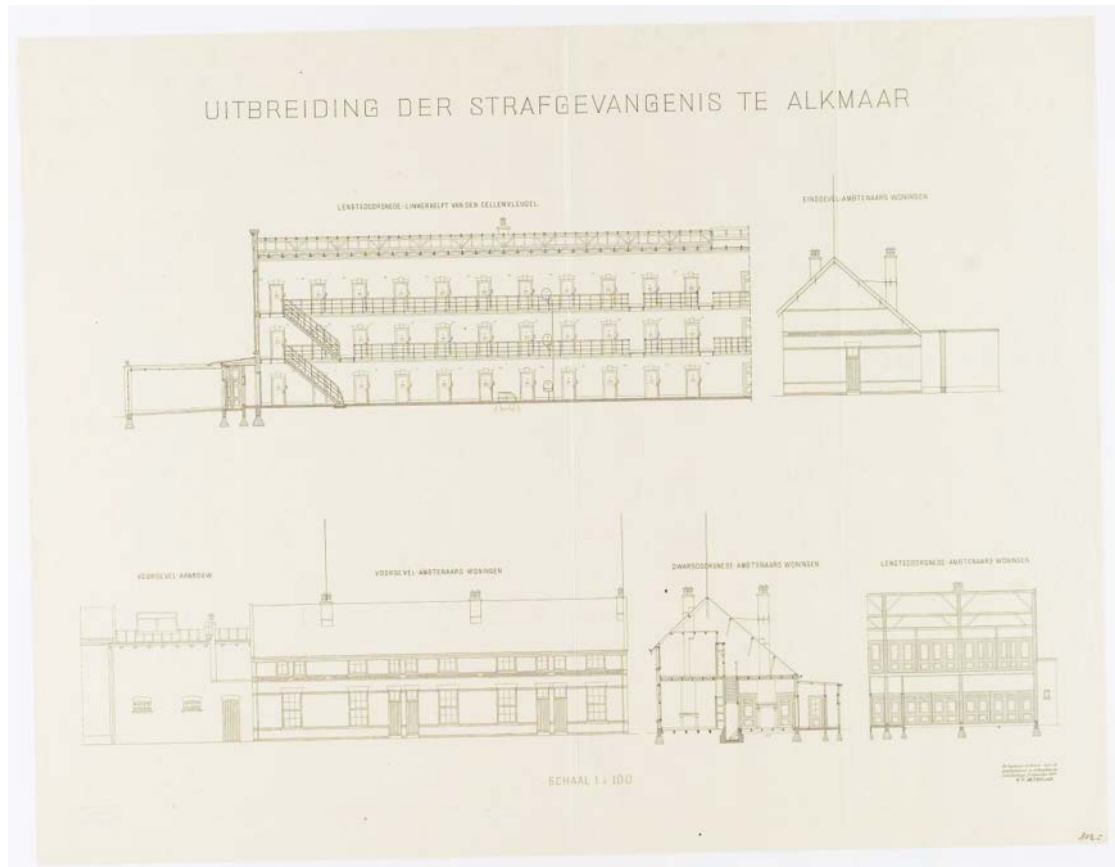
Bouwtekening uitbreiding W.C. Metzelaar september 1891 doorsneden (Regionaal Archief Alkmaar)
