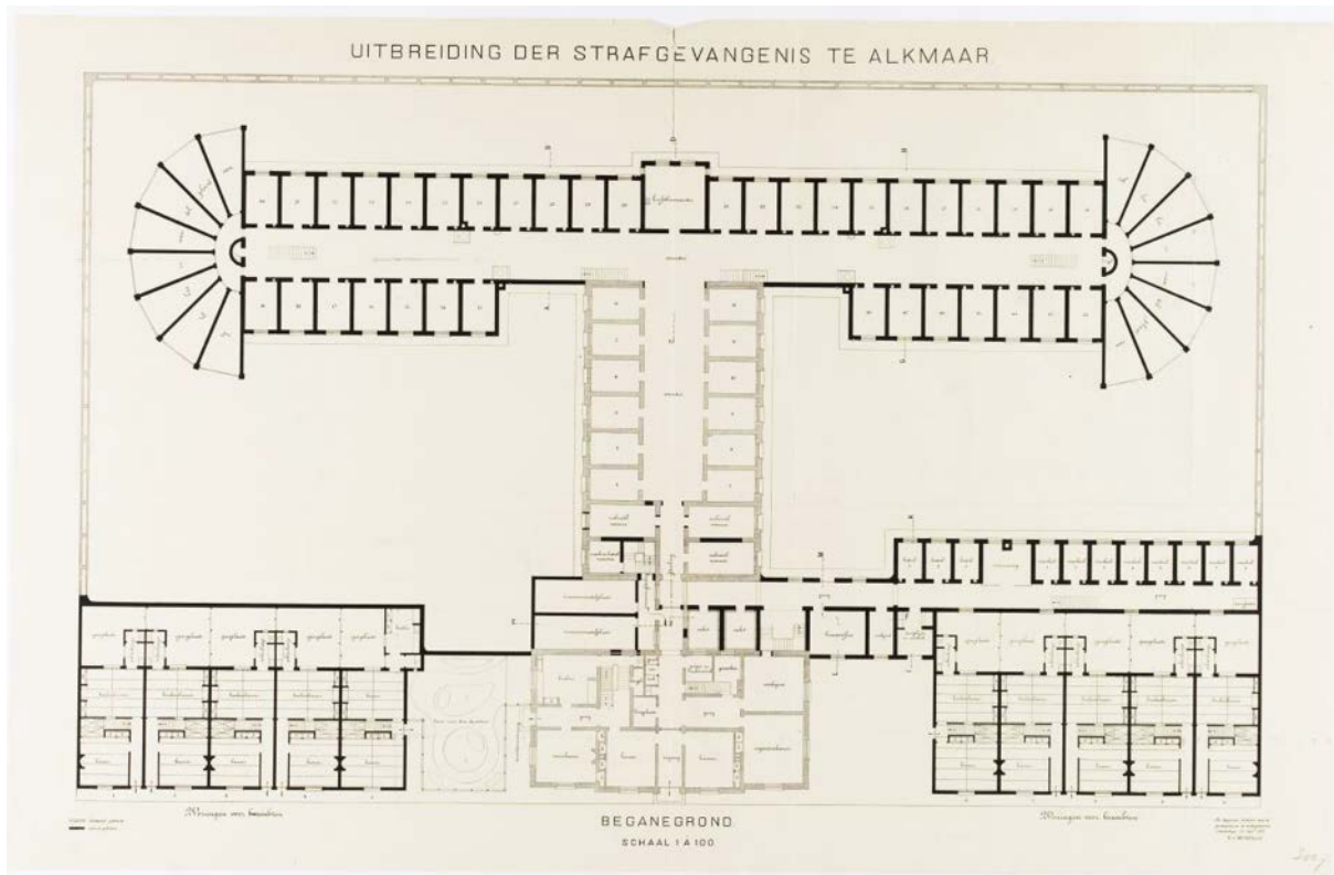
Bouwtekening uitbreiding W.C. Metzelaar september 1891 plattegrond begane grond. In lichtgrijs de oorspronkelijke gevangenis. In zwart de wijzigingen/uitbreidingen. (Regionaal Archief Alkmaar)
