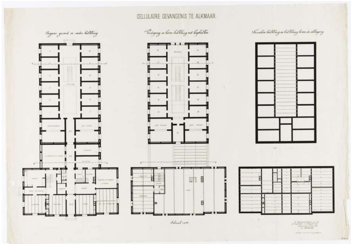
Bouwtekening J.F. Metzelaar juli 1883 plattegronden en balklagen (Regionaal Archief Alkmaar)
