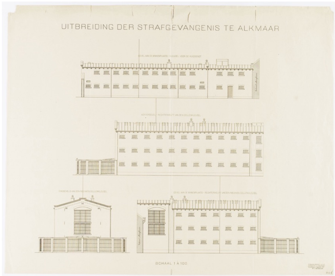
Bouwtekening uitbreiding W.C. Metzelaar september 1891 gevels (Regionaal Archief Alkmaar)
