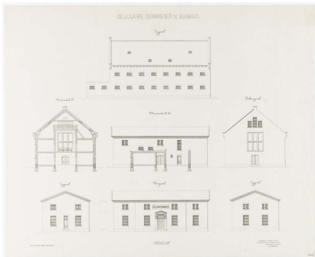
Bouwtekening J.F. Metzelaar juli 1883 gevels en doorsnede (Regionaal Archief Alkmaar)
