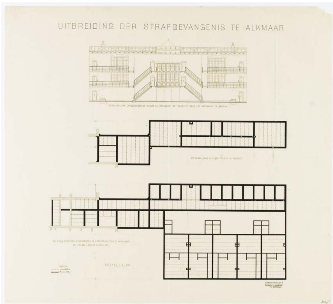
Bouwtekening uitbreiding W.C. Metzelaar september 1891 balklagen woningen & vleugel huisdienst gedeeltelijke langsddoorsnede nieuwe cellenvleugel (Regionaal Archief Alkmaar)
