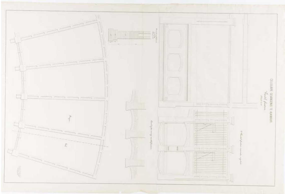
Bouwtekening J.F.Metzelaar juli 1883 wandplaats en regenbak (Regionaal Archief Alkmaar)
