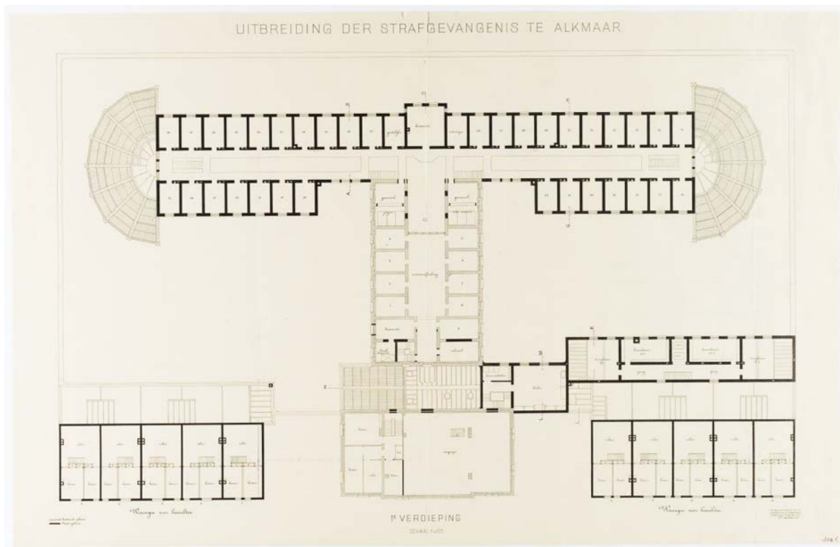
Bouwtekening uitbreiding W.C. Metzelaar september 1891 plattegrond eerste verdieping (Regionaal Archief Alkmaar)
