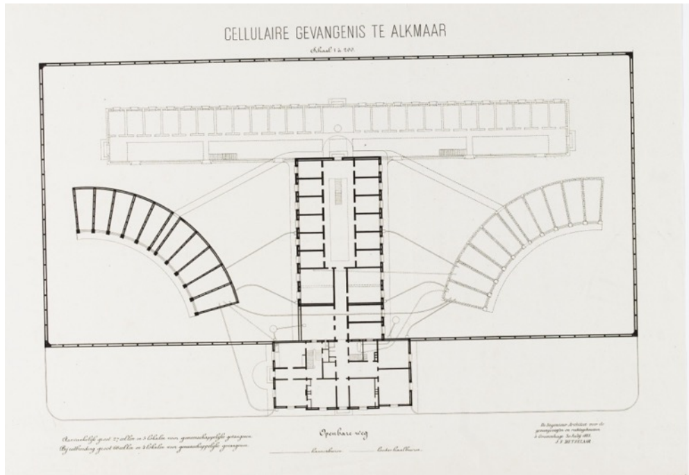
Bouwtekening J.F. Metzelaar juli 1883 plattegrond en beoogde uitbreiding (Regionaal Archief Alkmaar)
