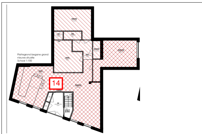
Wageweg 14 woning begane grond
